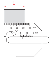
uzunluk ölçümü
