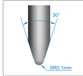
HSM5D uç
