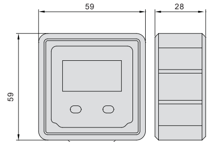
manyetik taban
