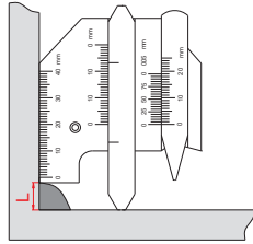
yükseklik ölçümü
